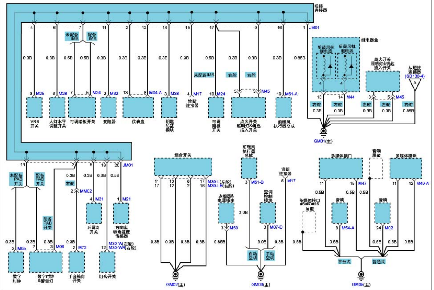
搭铁分布(3)
